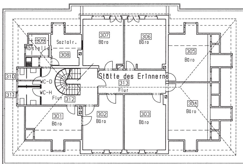
VILLA TEN HOMPEL DACHGESCHOSS
