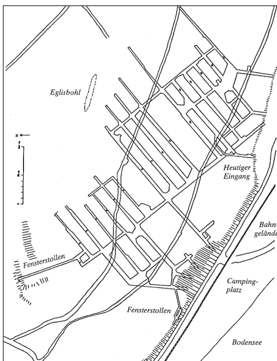
Plan des Überlingener Stollens. Zeichnung nach Plänen der Bundesanstalt für Bodenforschung. (aus: Oswald Burger, Der Stollen, Überlingen)
